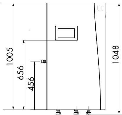
Frontansicht
