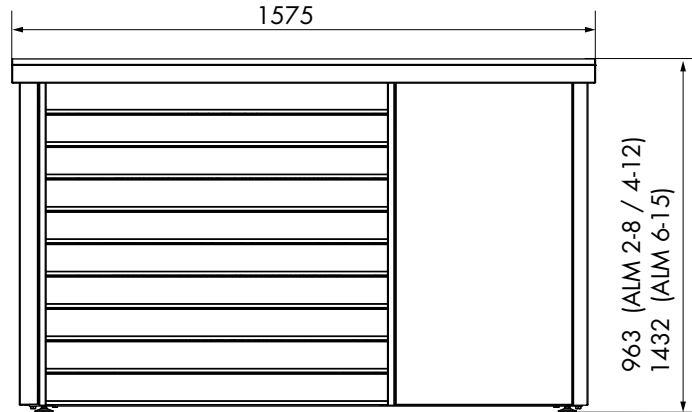
Frontansicht (Ausblasseite)
