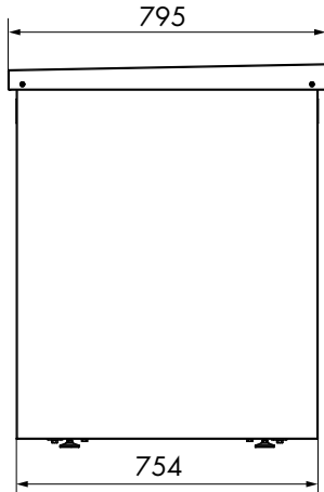
Seitenansicht rechts
