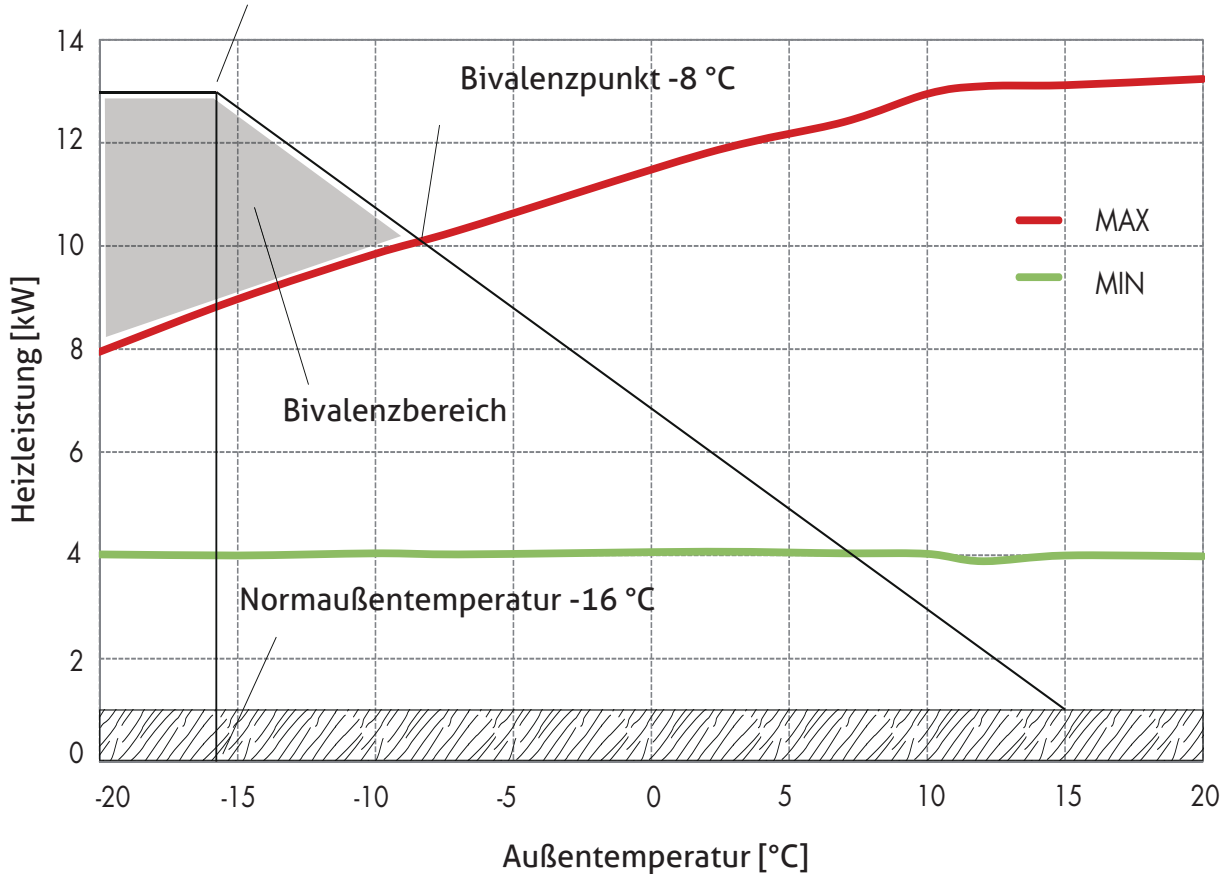
Benötigte Heizleistung von 13,2 kW bei Norm Aussentemperatur -16 °C Heizleistung inkl. Sperrzeitfaktor und Brauchwasserbedarf
